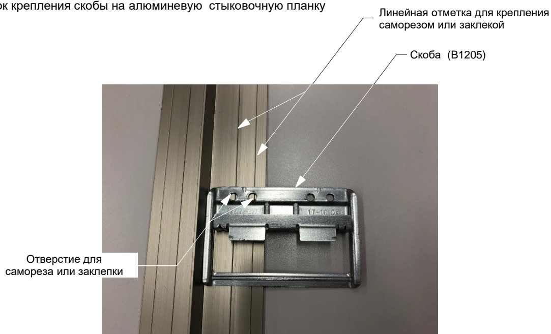
Т-образная алюминиевая стыковочная планка
